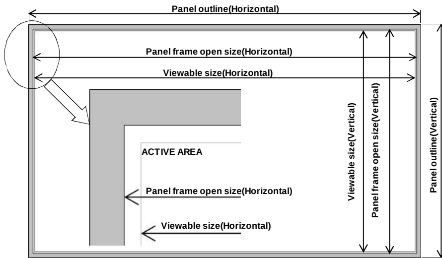
LCD Module
