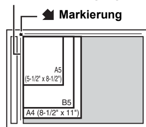
Skala des Vorlagenglasses
