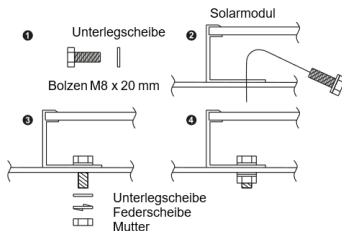
Abbildung 2. Komponenten für Schraubmontage
